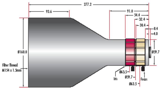
0.08X & 0.06X Telecentric Lens
