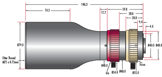
0.25X & 0.18X Telecentric Lenses
